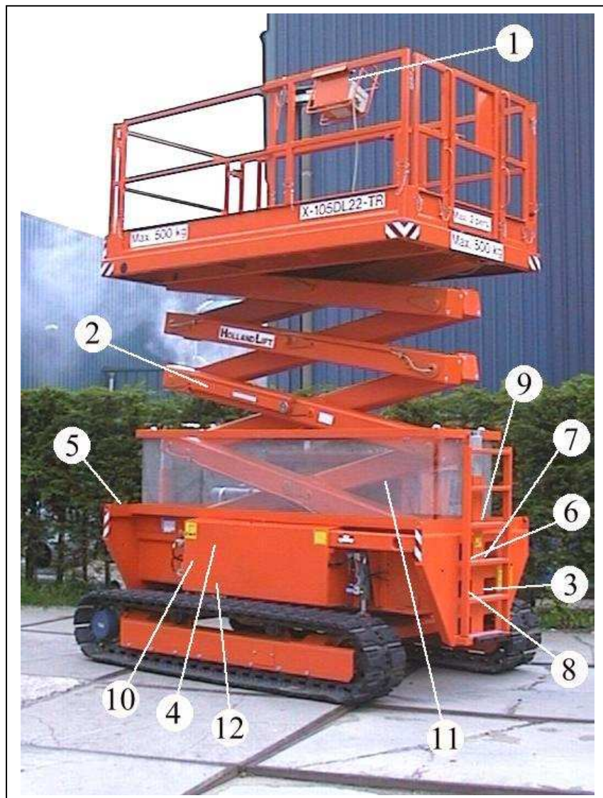
Afb. 5 Overzichtstekening veiligheidsvoorzieningen
