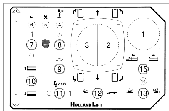
Afb. 18 Bedieningskast
