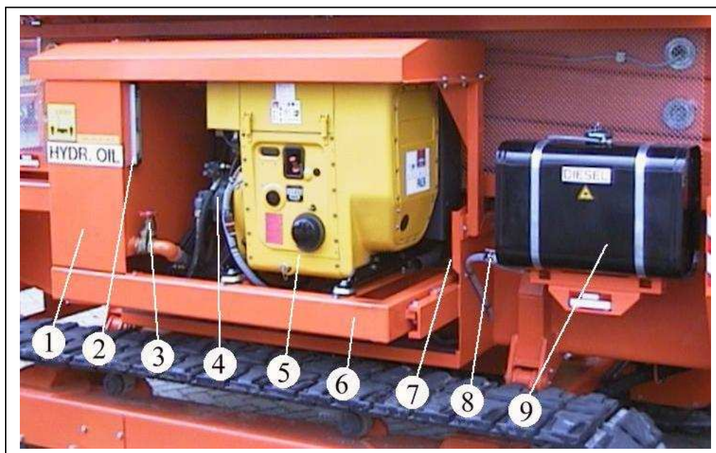
Afb. 15 Dieselmotor
