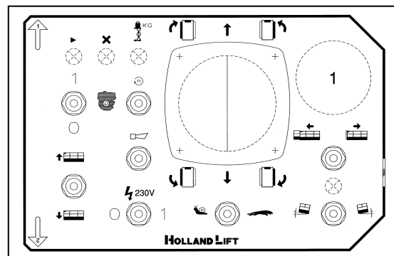
Afb. 6 Bedieningskast
