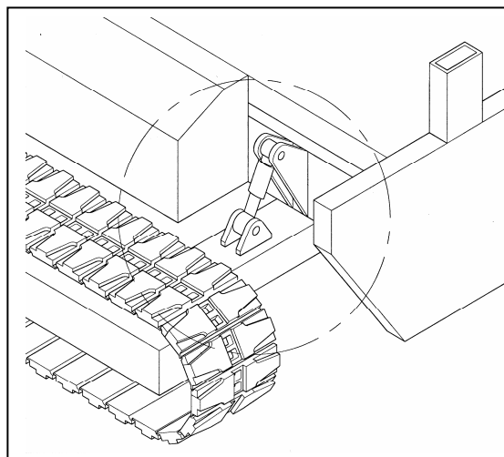
Afb. 14 Nivelleercilinder
