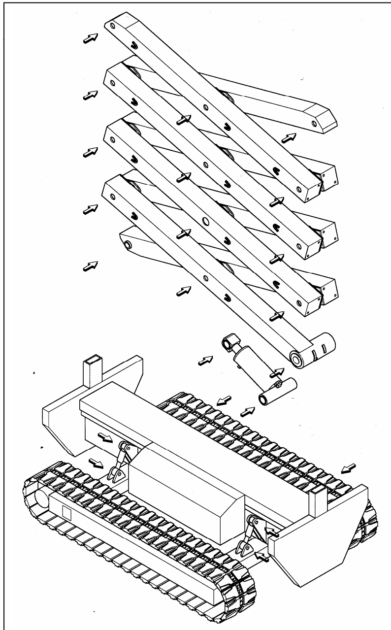
Afb. 24 Overzicht smeerpunten
