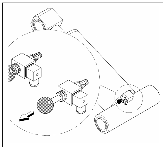
Afb. 9 Nooddaalvoorziening
