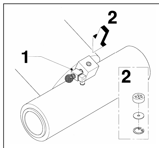
Afb. 10 Leiding-/slangbreukbeveiliging
