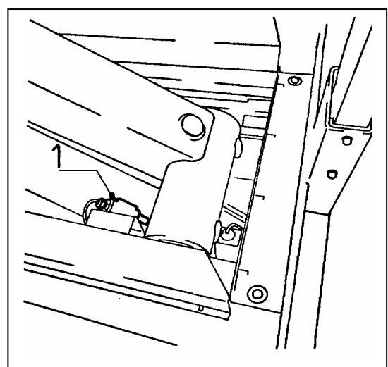
Afb. 8 Eindschakelaar hefcilinder 1. Eindschakelaar
